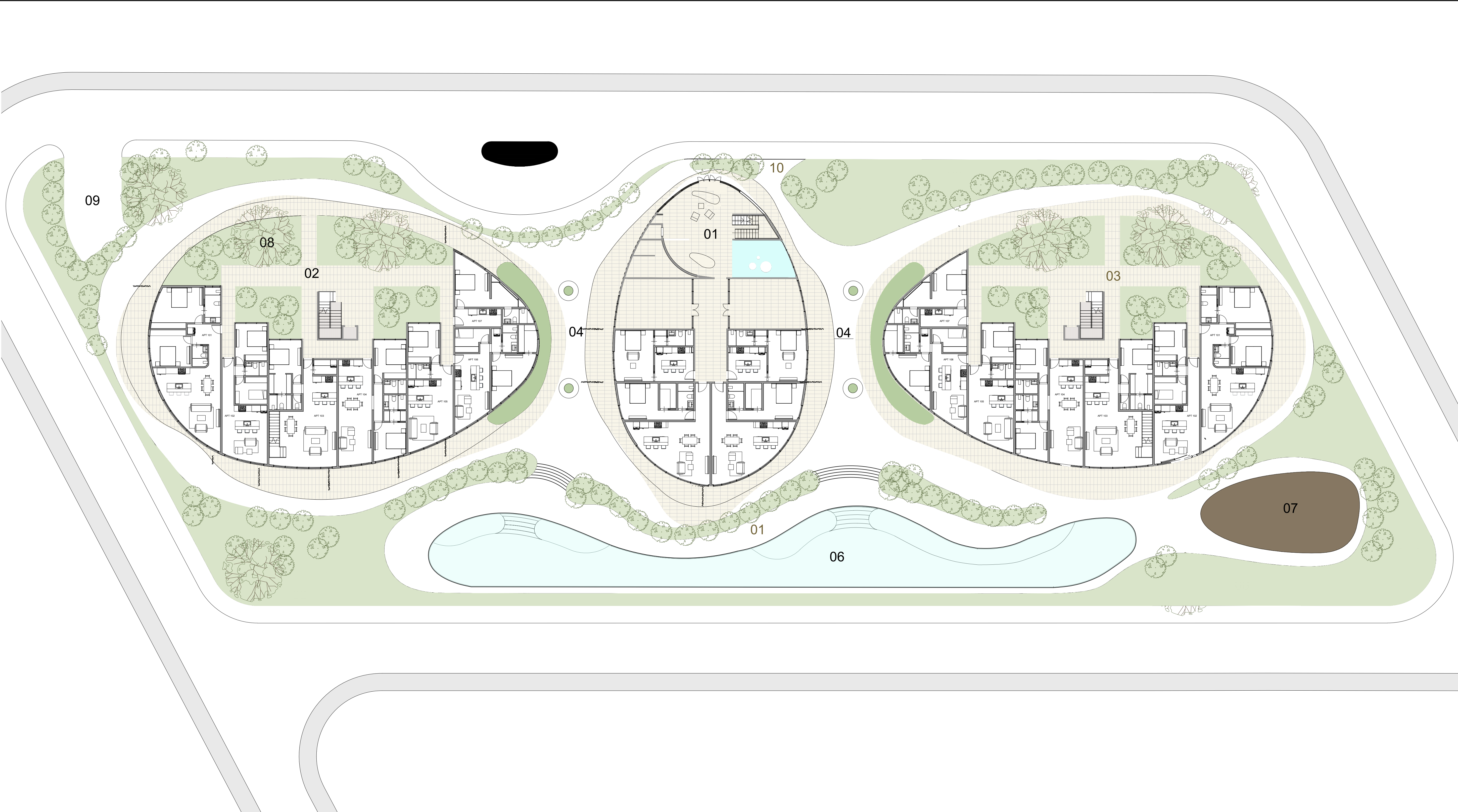
1 PLANTA ARQUITECTONICA DE MASTER PLAN 1ER NIVEL 1 : 200
