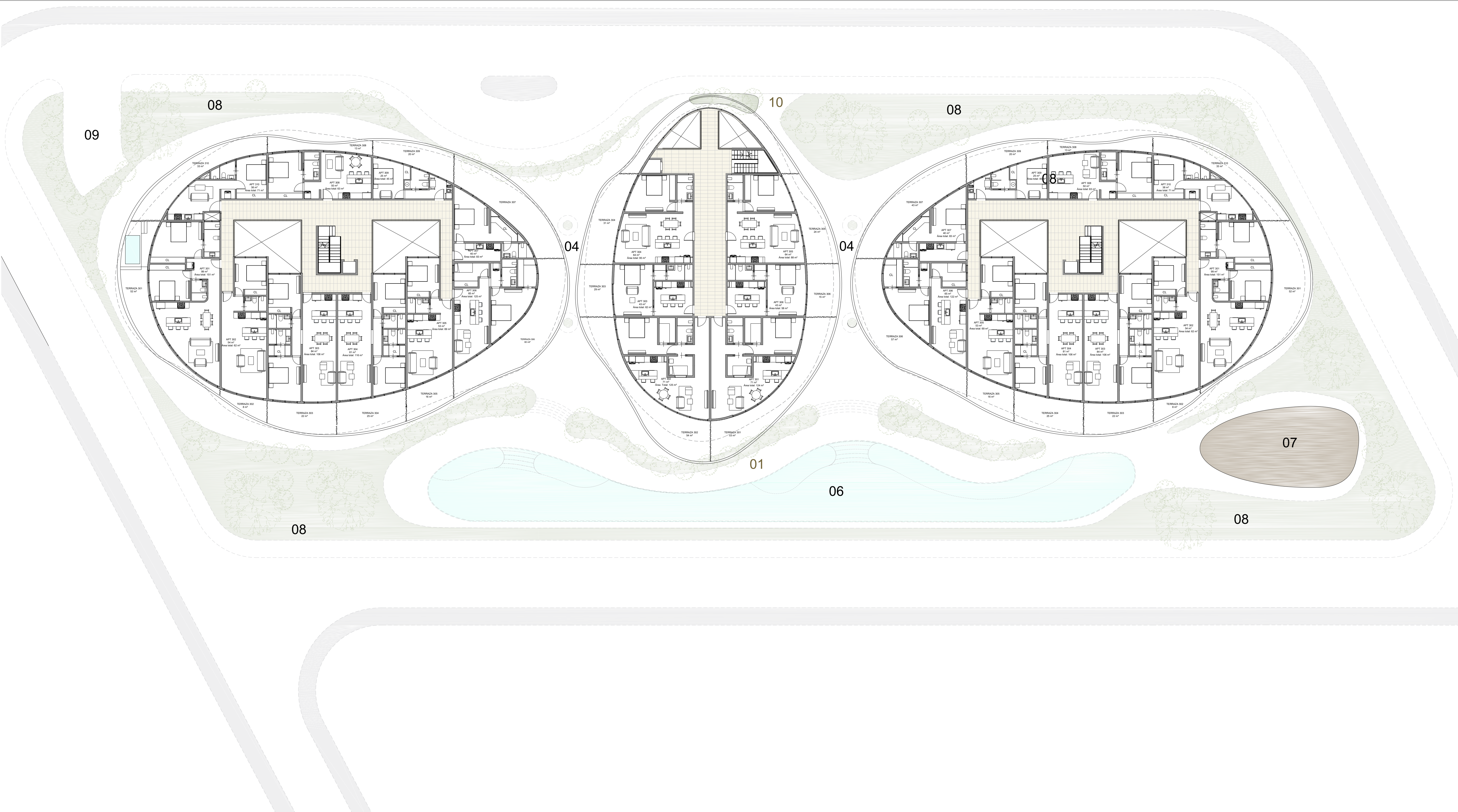
1 PLANTA ARQUITECTONICA DE MASTER PLAN 3ER NIVEL 1 : 200
