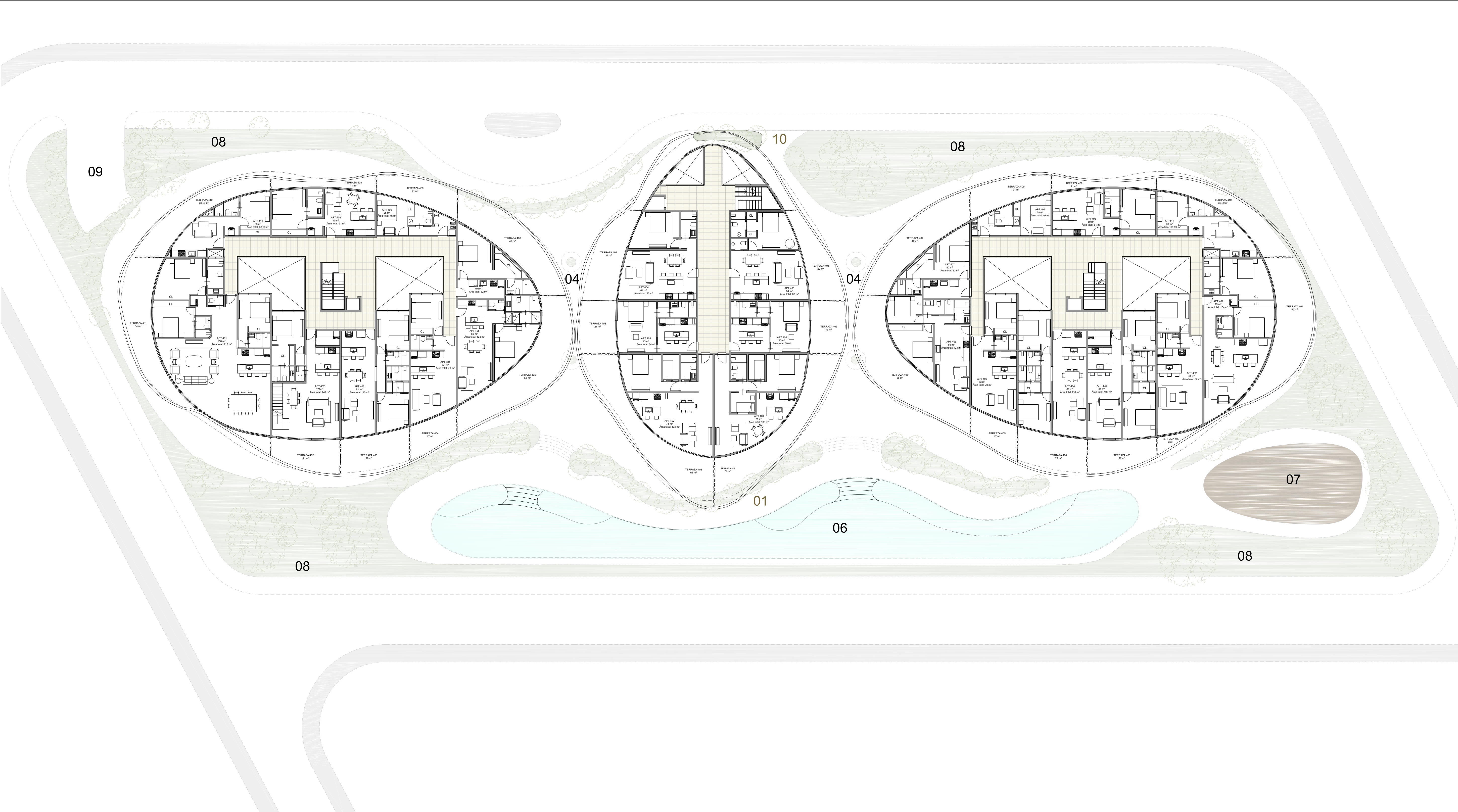
1 PLANTA ARQUITECTONICA DE MASTER PLAN 4TO NIVEL 1 : 200
