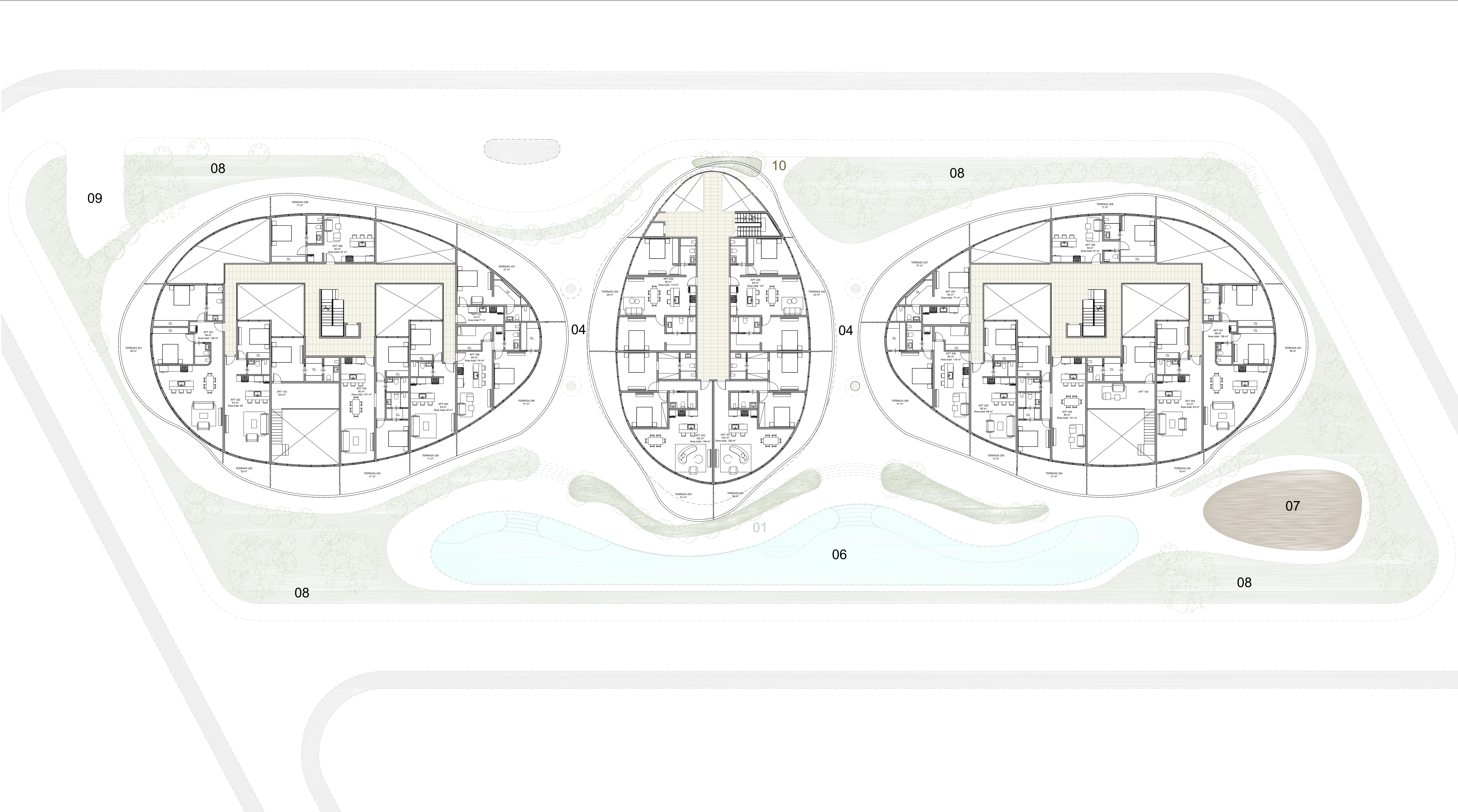
1 PLANTA ARQUITECTONICA DE MASTER PLAN 2DO NIVEL 1 : 200
